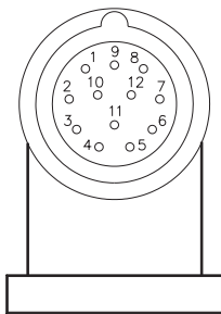
Vue de devant connecteur Résolveur
