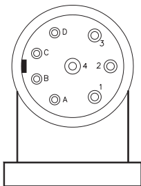
Vue de devant connecteur de puissance
